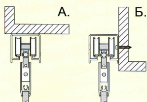
Профиль горизонтальный SEZAM
